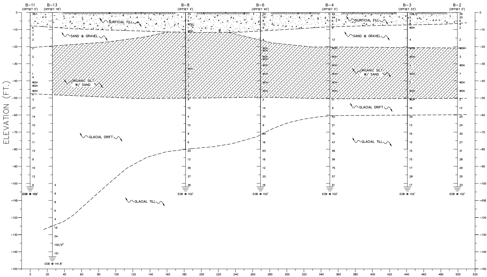
CROSS SECTION B-B' HORIZ. SCALE: 1" = 20' VERT. SCALE: 1" = 10'
